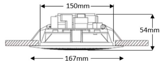
TI-CS4 - Dimensions
