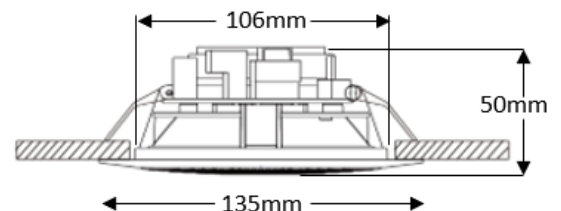
TI-CS3 - Dimensions
